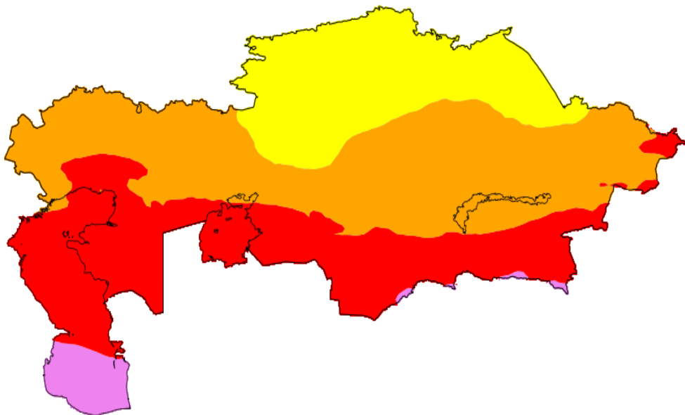
Рис. Распределение УФ индекса по территории Казахстана 03 июля 2020 г.
