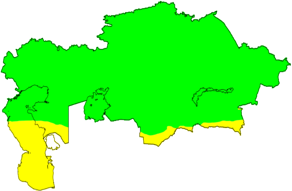
Рис. Распределение УФ индекса по территории Казахстана 25 сентября 2020 г.
