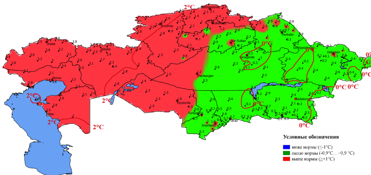
Фактическое отклонение температуры воздуха от нормы в июле 2020 года
