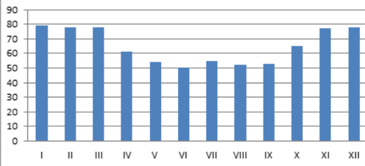
Средняя месячная относительная влажность воздуха, % г. Караганда
