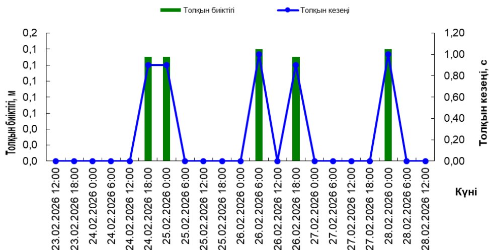
21050 квадратындағы толқындар
