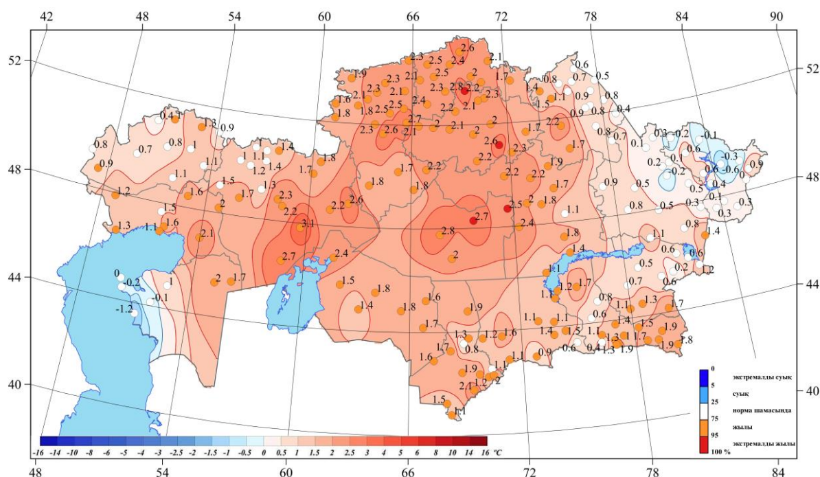
2 – сурет. 1991–2020 жылдардағы кезеңге қатысты есептелген 2026 жылғы мамыр айындағы орташа айлық ауа температурасы (°C) аномалияларының кеңістіктік таралуы және 1941–2026 жылдардағы кезеңге сәйкес есептелген ауа температурасының аспау ықтималдығының кеңістіктік таралуы
