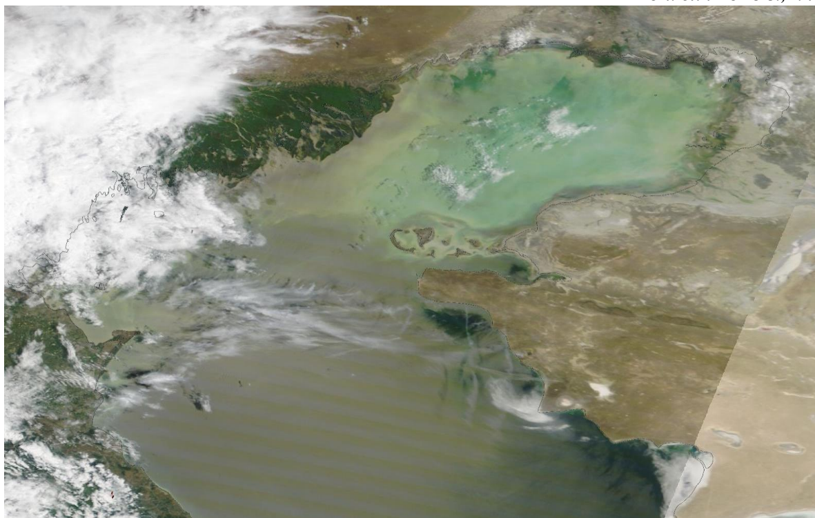
Рис.1 Космический снимок Каспийского моря, 06 июля, 2026 г. NASA/GSFC
