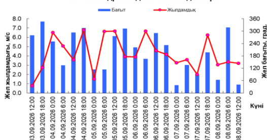
21142 квадратындағы жел жағдайлары
