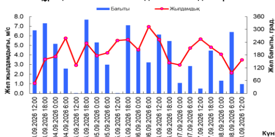
Құрық шығанағы аймағындағы жел жағдайлары
