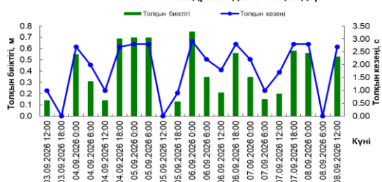
21141 квадратындағы толқындар
