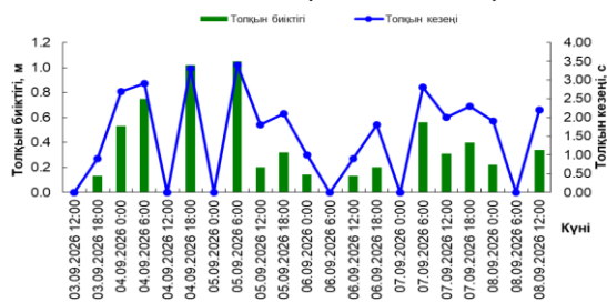
21050 квадратындағы толқындар
