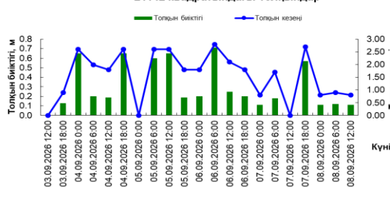
21142 квадратындағы толқындар
