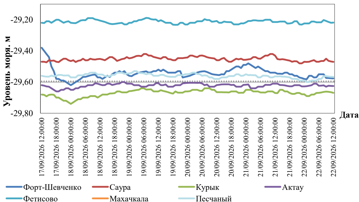
Рис.2 Прогноз уровня моря в пунктах Среднего Каспия
