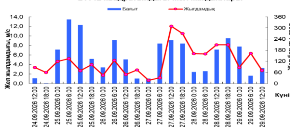
21142 квадратындағы жел жағдайлары
