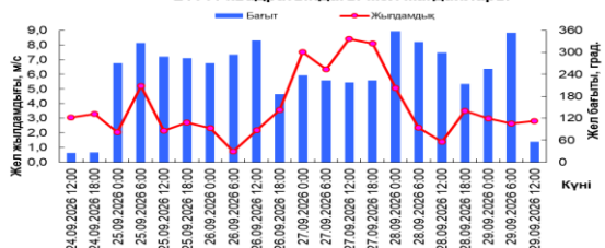
21141 квадратындағы жел жағдайлары
