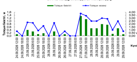
21142 квадратындағы толқындар
