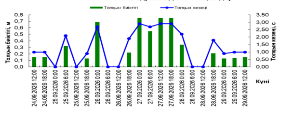
21141 квадратындағы толқындар
