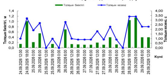
21050 квадратындағы толқындар
