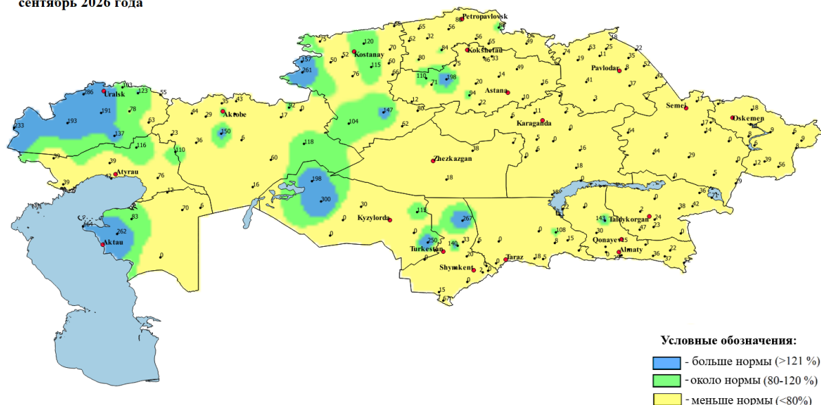
Аномалия количества осадков за сентябрь 2026 года
