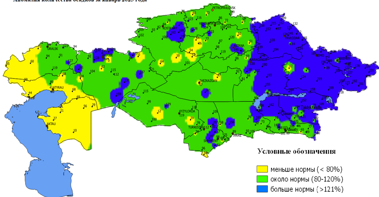
Аномалия количества осадков за январь 2023 года
