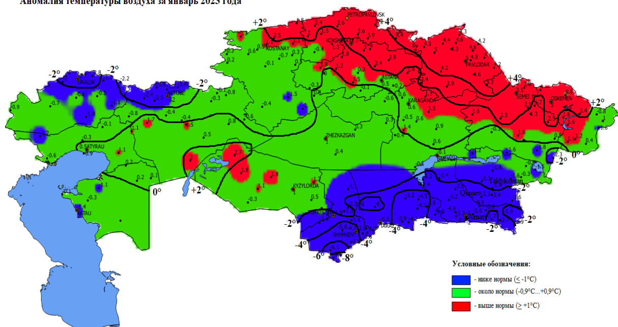
Аномалия температуры воздуха за январь 2023 года
