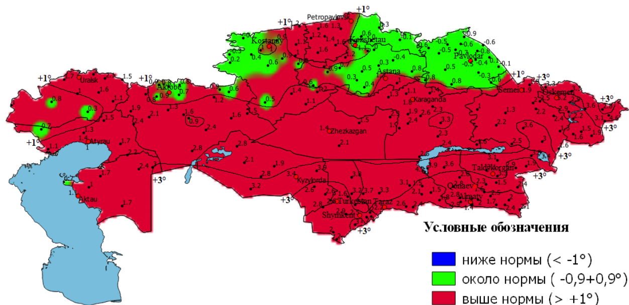
Аномалия температуры воздуха за февраль 2023 года
