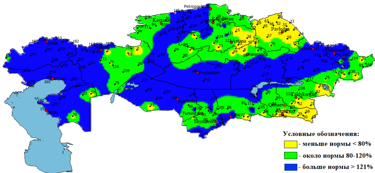
Аномалия количества осадков за февраль 2023 года
