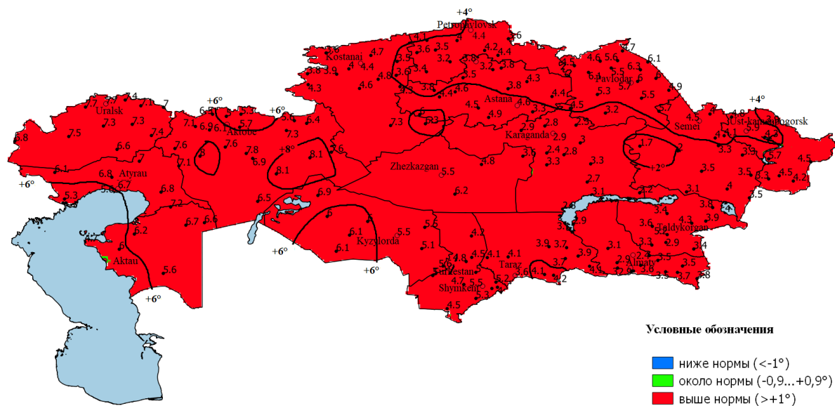
Аномалия температуры воздуха за март 2023 года
