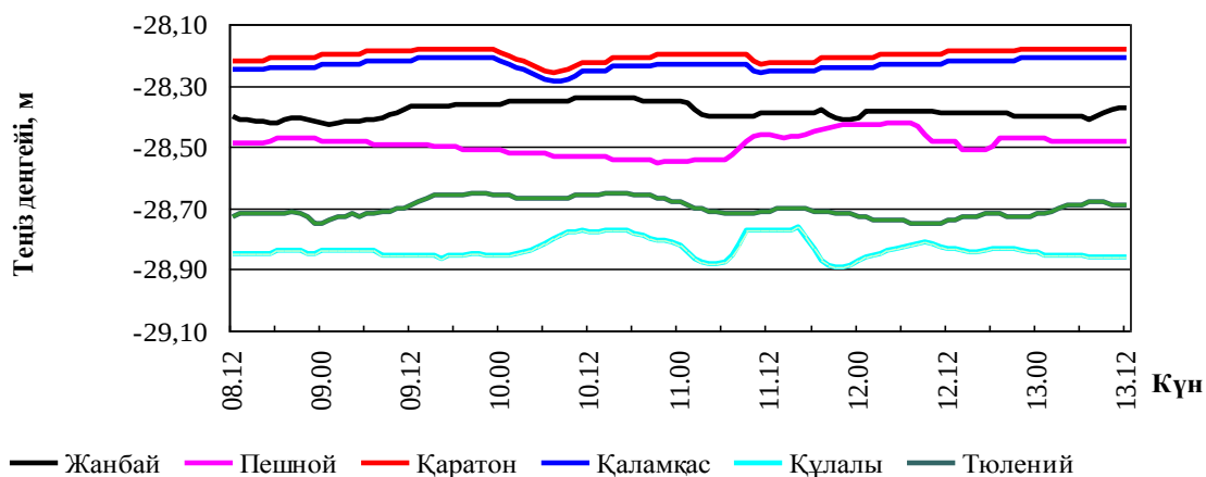
2-сурет. Солтүстік Каспийдегі теңіз деңгейінің болжамы
