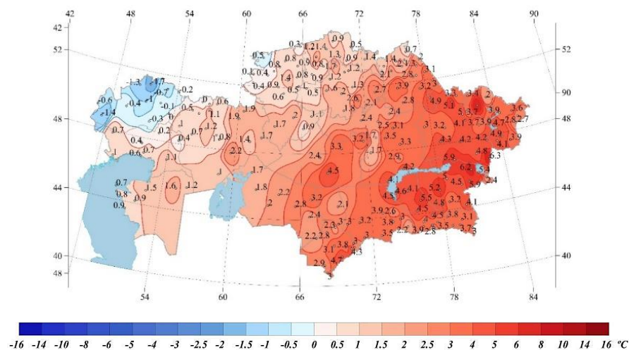
Рисунок 1 – Пространственное распределение аномалий средней месячной температуры воздуха (°С) в январе 2024 г., рассчитанных относительно норм за период 1991-2020 гг.
