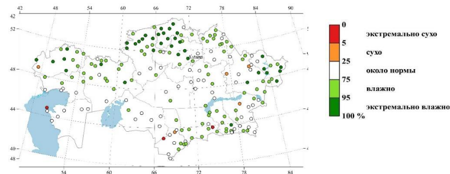
Рисунок 4 – Пространственное распределение вероятности не превышения количества атмосферных осадков января 2024 г. Вероятности рассчитаны по данным периода 1941-2024 гг.
