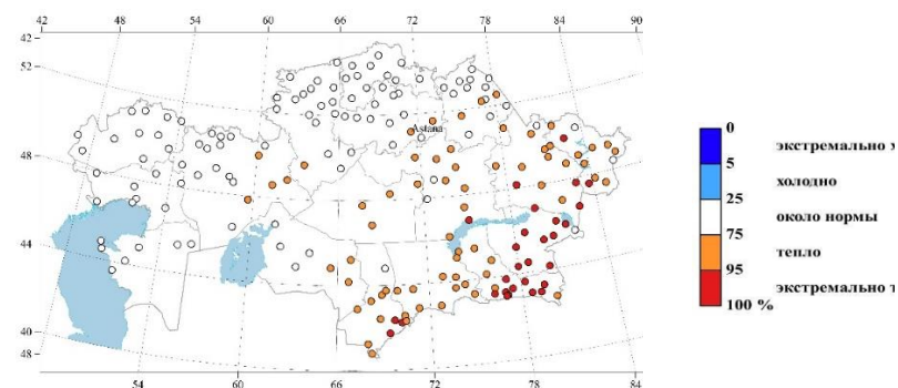
Рисунок 2 – Пространственное распределение вероятностей непревышения температуры воздуха в январе 2024 г., рассчитанных по данным периода 1941-2024 гг.
