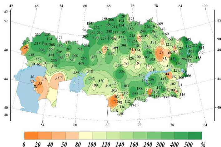
Рисунок 3 – Пространственное распределение количества атмосферных осадков в январе 2024 г. (в % нормы, рассчитанной относительно базового периода 1991-2020 гг.)
