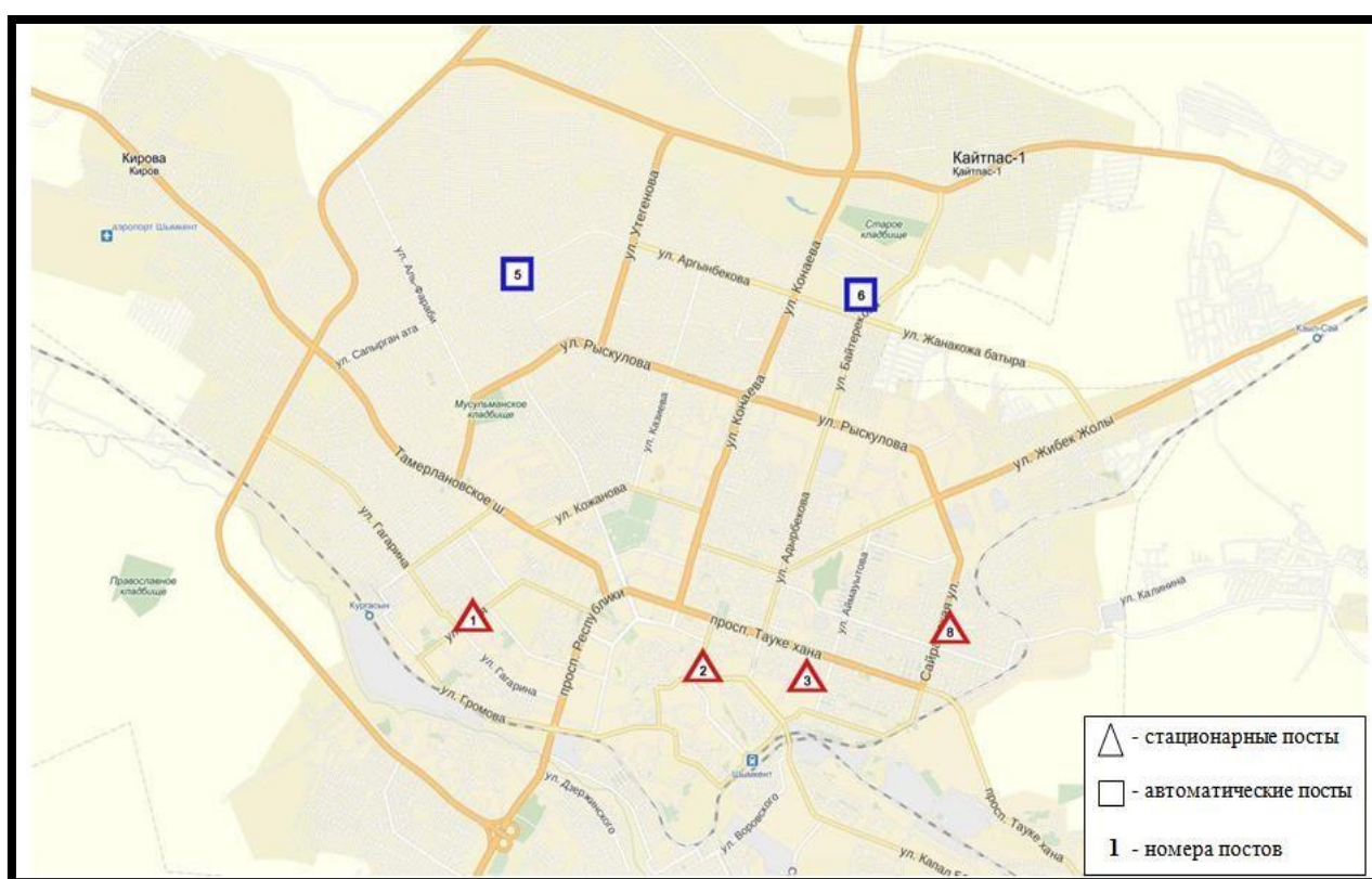
Рис 1 Схема расположения стационарной сети наблюдения за загрязнением атмосферного воздуха г.Шымкент
