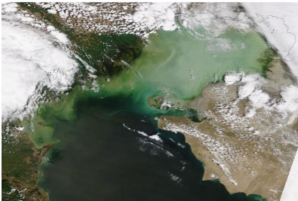
2024 ж. 27 маусым ғарыштан түсірілген Каспий теңізінің солтүстік бөлігінің суреті («NASA» жобасының суреті)
