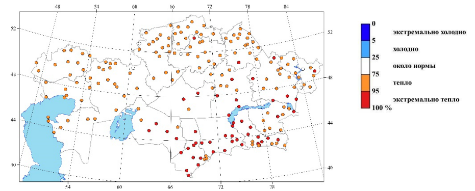
Рисунок 2 – Пространственное распределение вероятностей не превышения температуры воздуха в июне 2024 г., рассчитанных по данным периода 1941-2024 гг.
