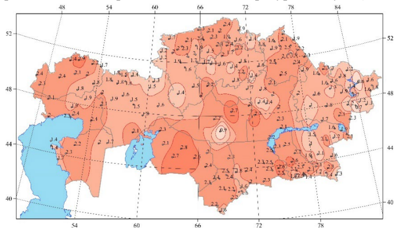
Рисунок 1 – Пространственное распределение аномалий средней месячной температуры воздуха (°С) в июне 2024 г., рассчитанных относительно норм за период 1991-2020 гг.
