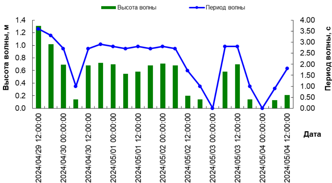
Волнение в квадрате 21141
