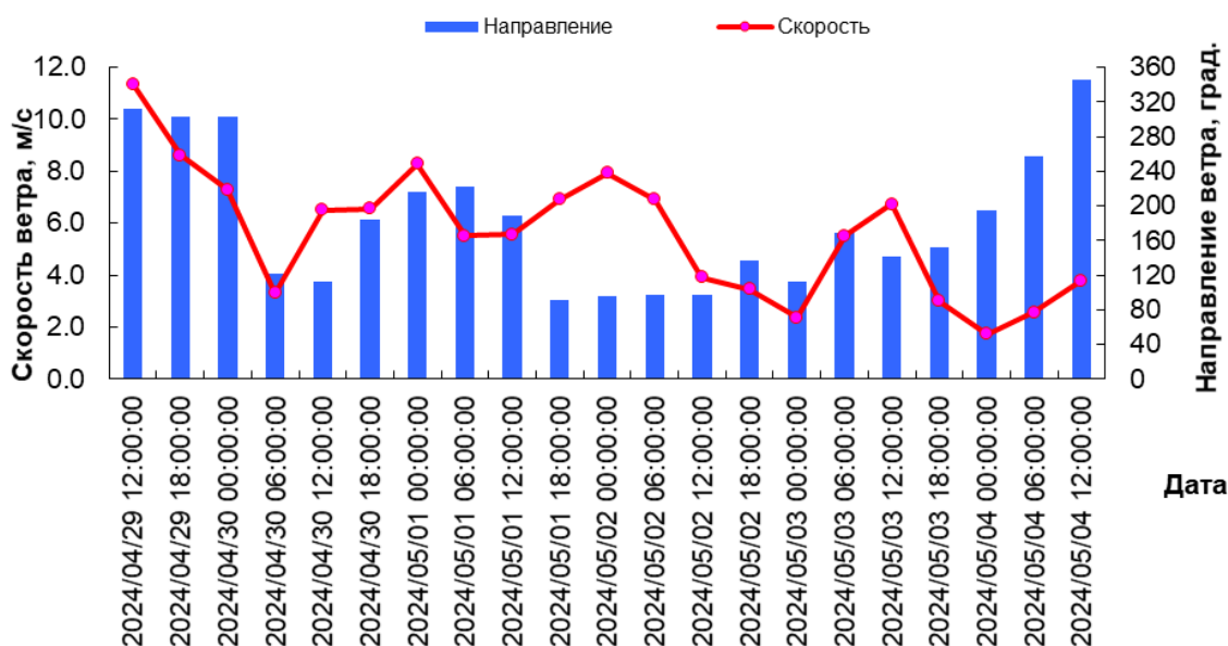
Ветровые условия в квадрате 21141
