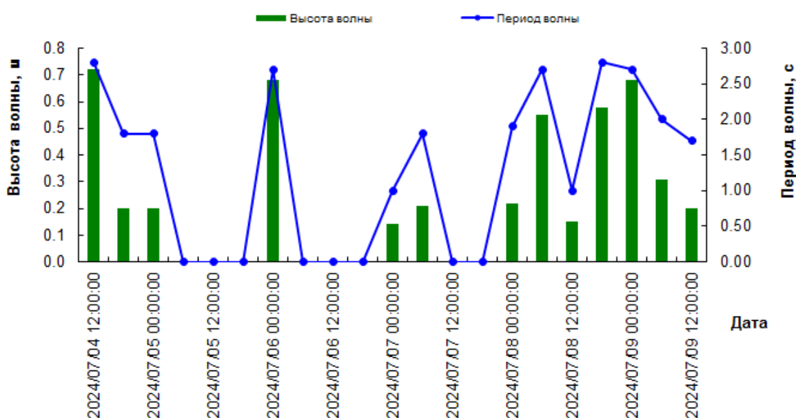
Волнение в квадрате 21141
