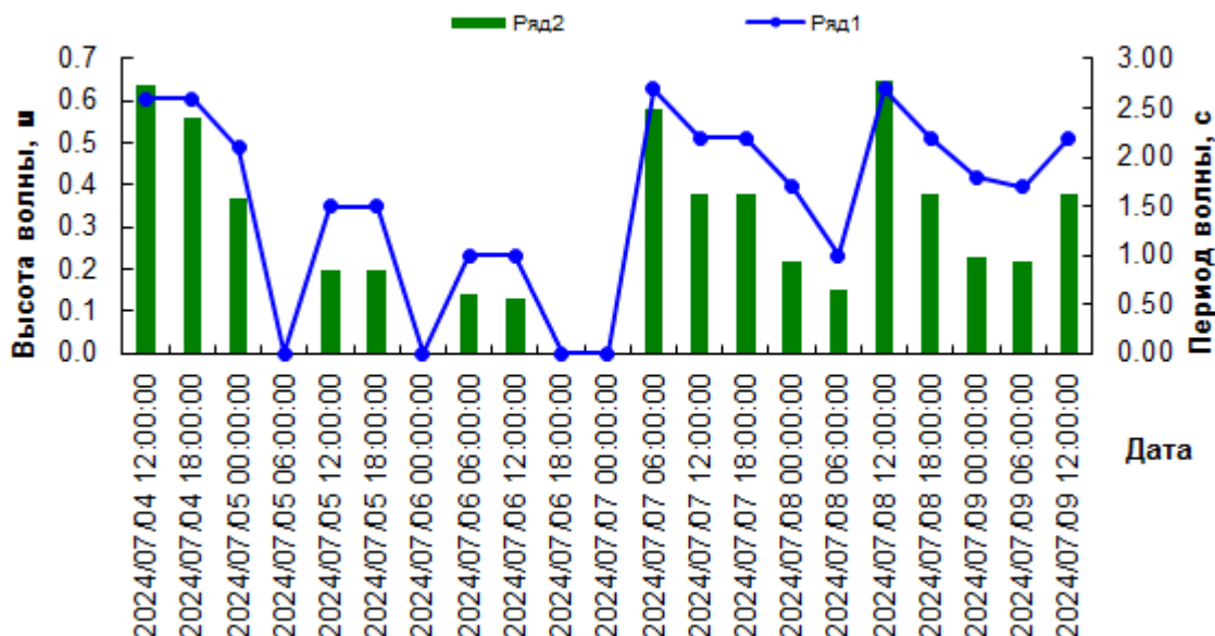
Волнение в квадрате 21050
