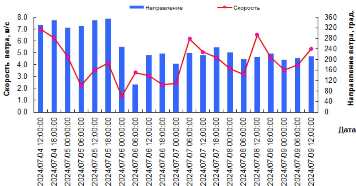
Ветровые условия в квадрате 21050
