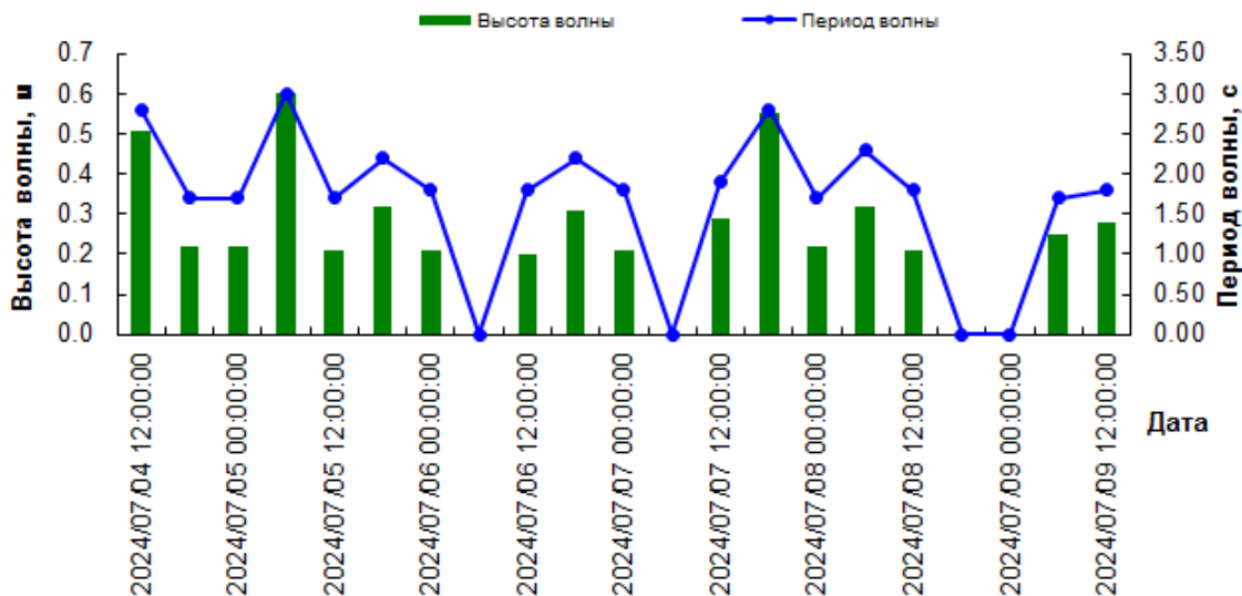
Волнение в бухте Курык
