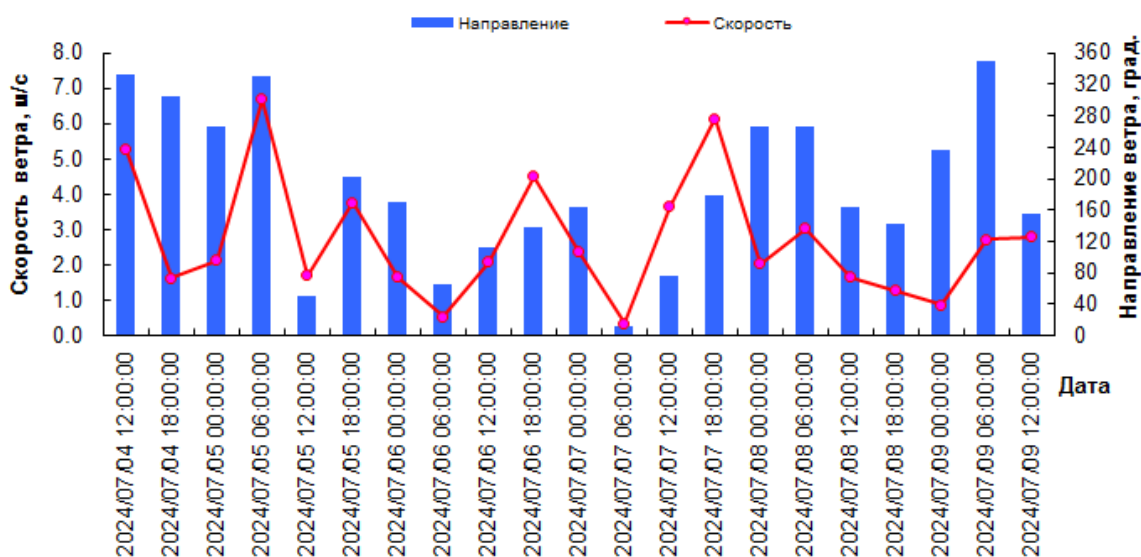
Ветровые условия в бухте Курык
