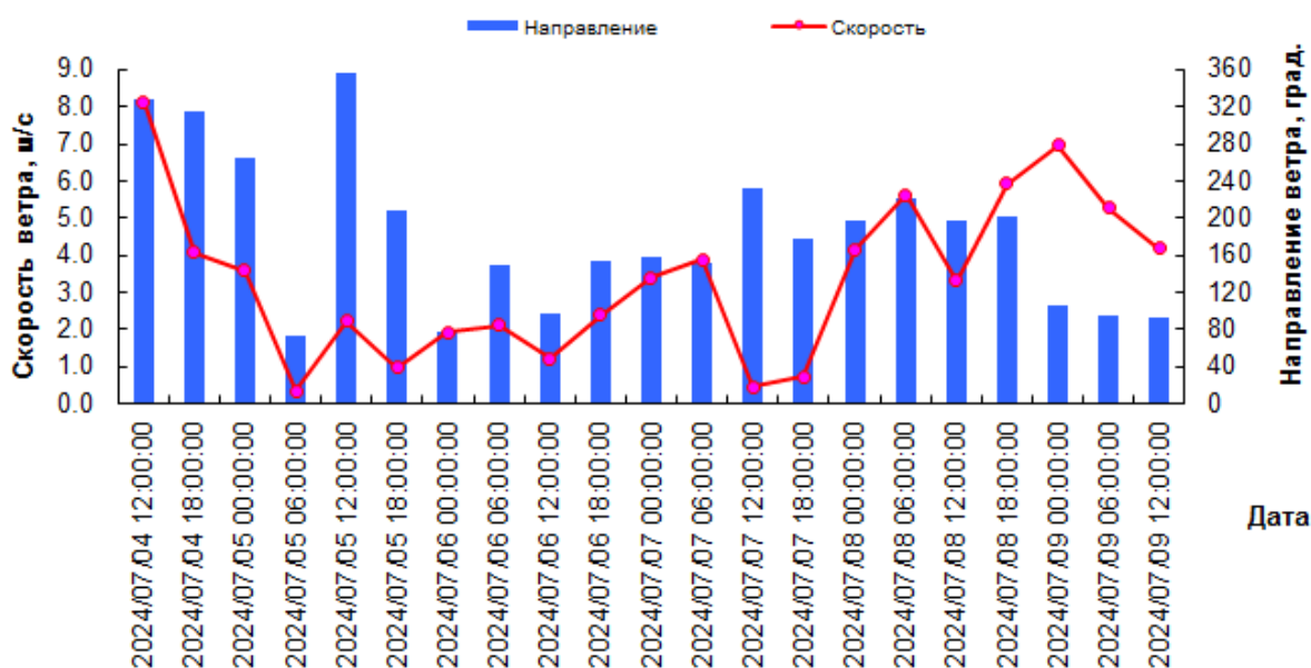
Ветровые условия в квадрате 21141
