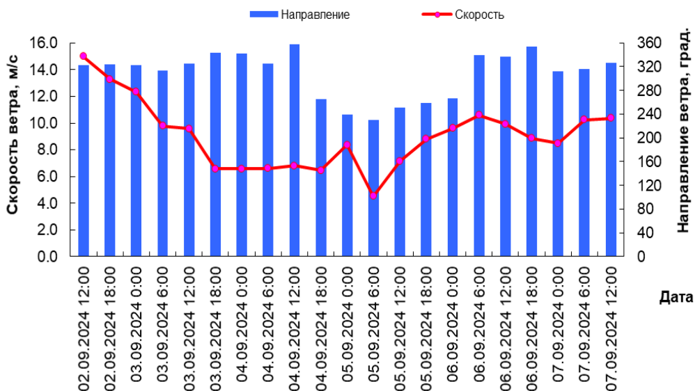
Ветровые условия в квадрате 21050
