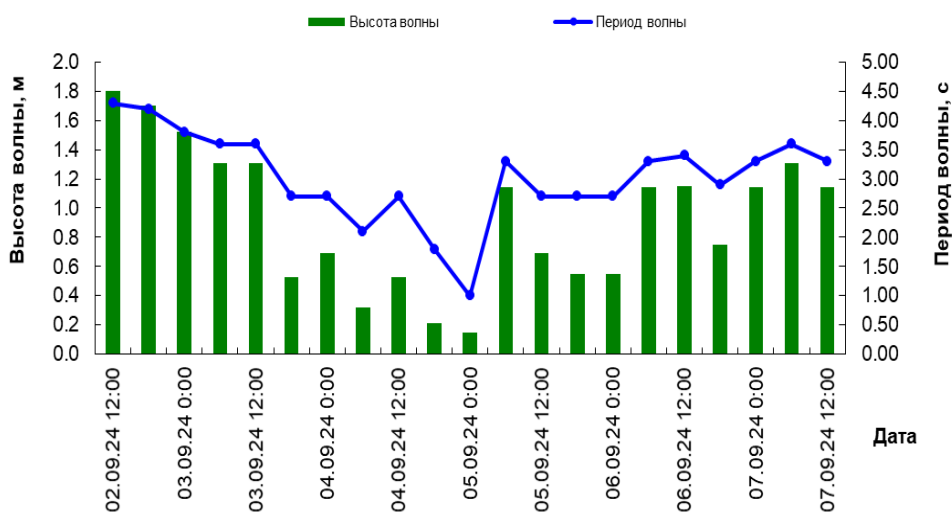
Волнение в квадрате 21141
