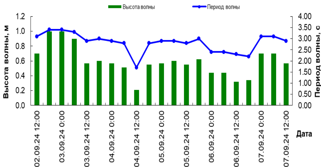
Волнение в бухте Курык
