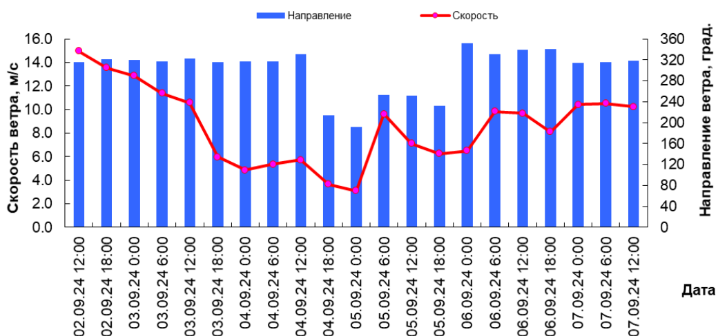
Ветровые условия в квадрате 21141
