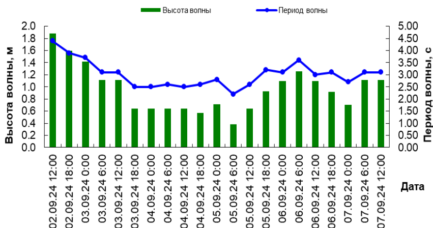
Волнение в квадрате 21050
