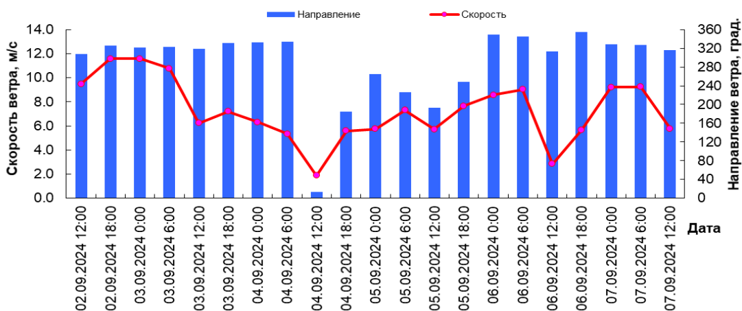
Ветровые условия в бухте Курык
