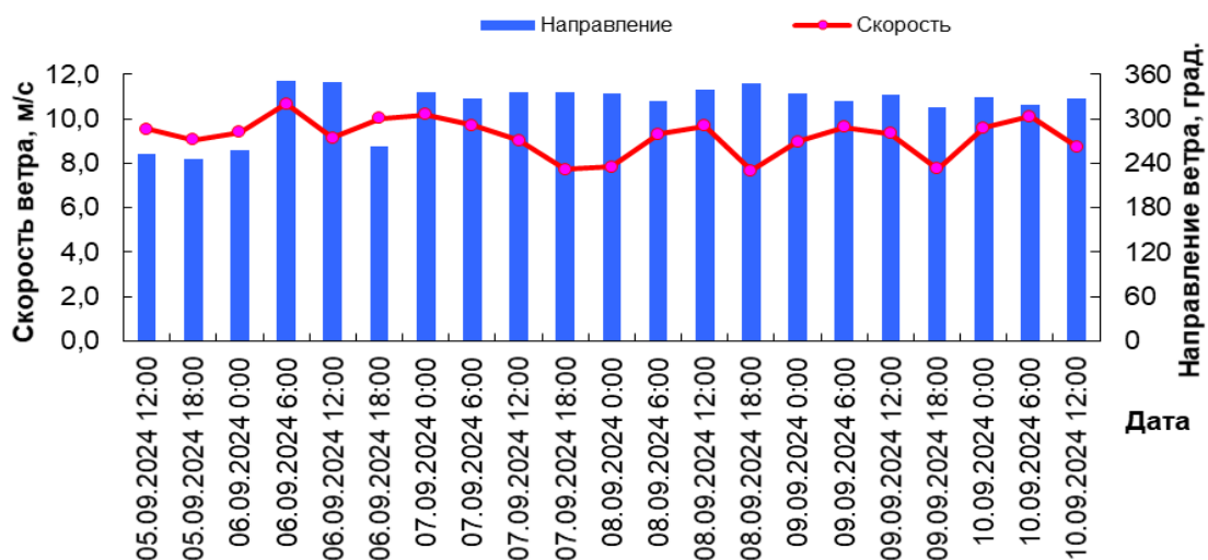
Ветровые условия в квадрате 21050
