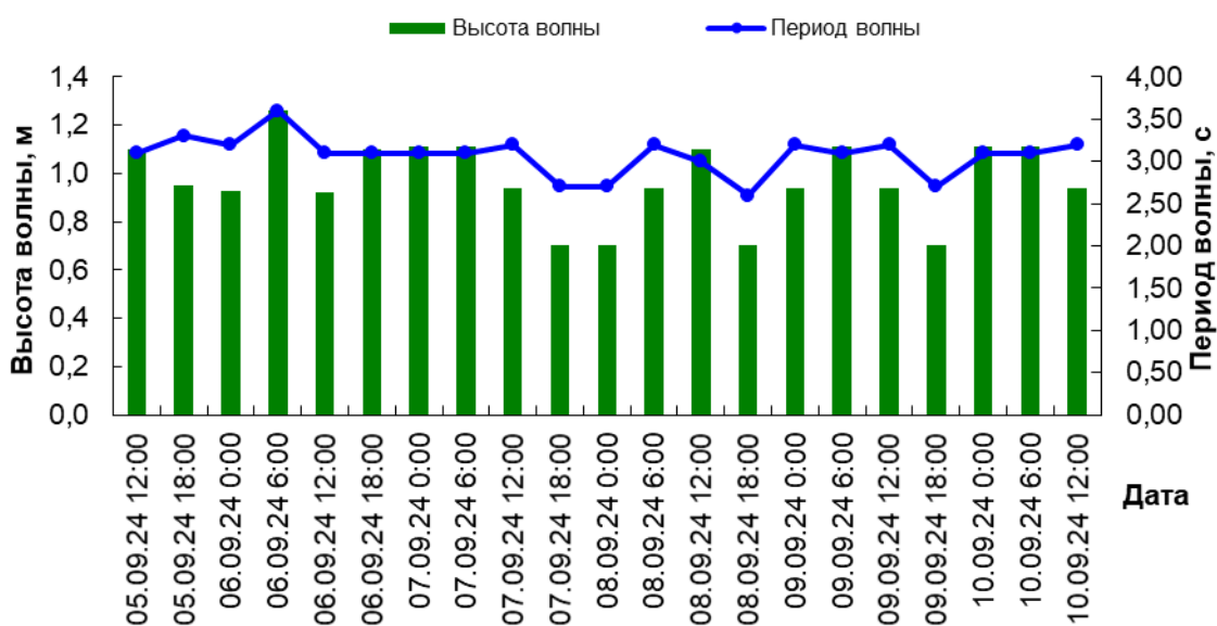
Волнение в квадрате 21050
