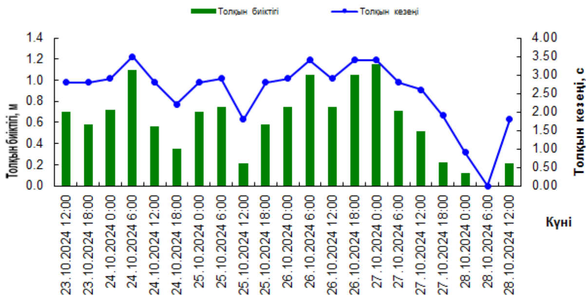
21050 квадратындағы толқындар
