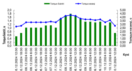
21050 квадратындағы толқындар
