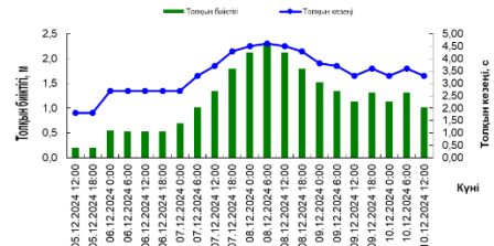
21141 квадратындағы толқындар
