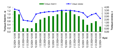
Баутино шығанағы аймағындағы толқындар
