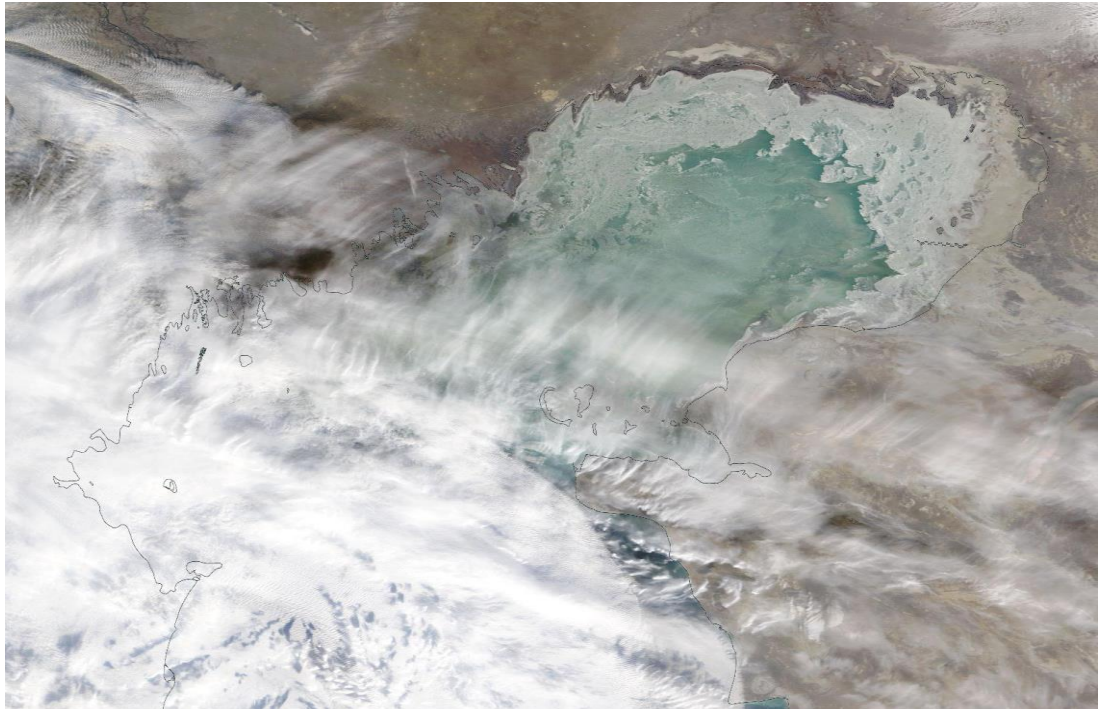
Каспий теңізінің ғарыштық суреті, 27 желтоқсан 2024 ж. (NASA/GSFC)
