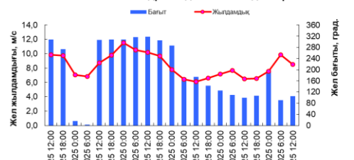
21142 квадратындағы жел жағдайлары
