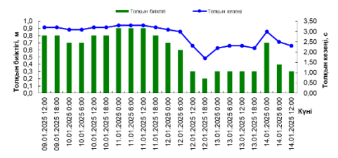
Баутино шығанағы аймағындағы толқындар
