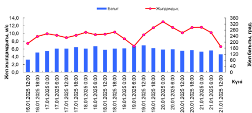
21050 квадратындағы жел жағдайлары
