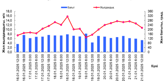
Құрық шығанағы аймағындағы жел жағдайлары
