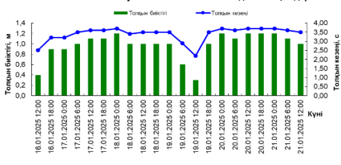
Баутино шығанағы аймағындағы толқындар
