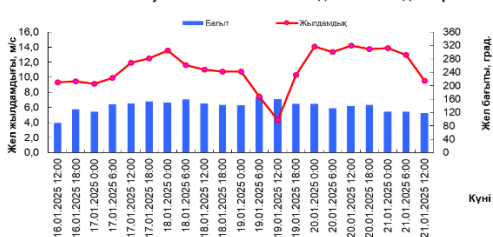
Баутино шығанағы аймағындағы жел жағдайлары
