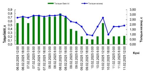
21050 квадратындағы толқындар
