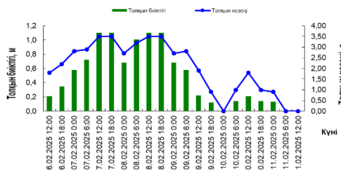
21141 квадратындағы толқындар
