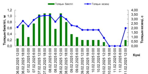
21142 квадратындағы толқындар
