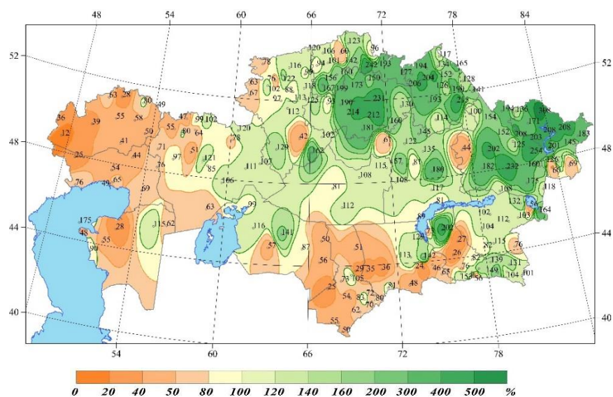
Рисунок 3 – Пространственное распределение количества атмосферных осадков в январе 2025 г. (в % нормы, рассчитанной относительно базового периода 1991-2020 гг.)
