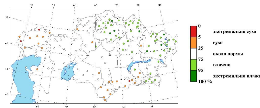
Рисунок 4 – Пространственное распределение вероятности непревышения количества атмосферных осадков в январе 2025 г. Вероятности рассчитаны по данным периода 1941-2025 гг.
