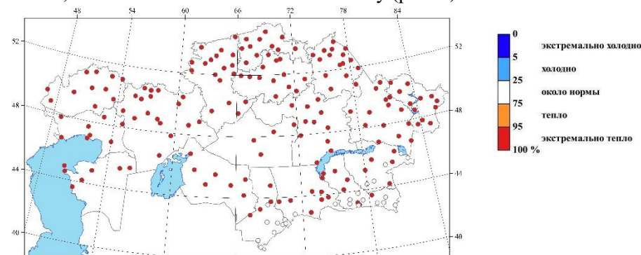
Рисунок 2 – Пространственное распределение вероятностей превышения температуры воздуха в январе 2025 г., рассчитанных по данным периода 1941-2025 гг.
