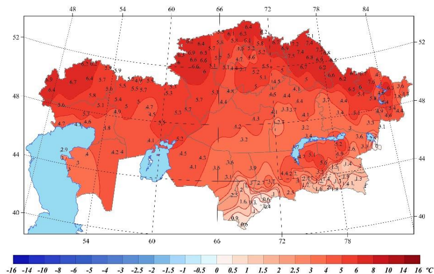
Рисунок 1 – Пространственное распределение аномалий средней месячной температуры воздуха ( ^{\circ}\text{C} ) в январе 2025 г., рассчитанных относительно норм за период 1991-2020 гг.
