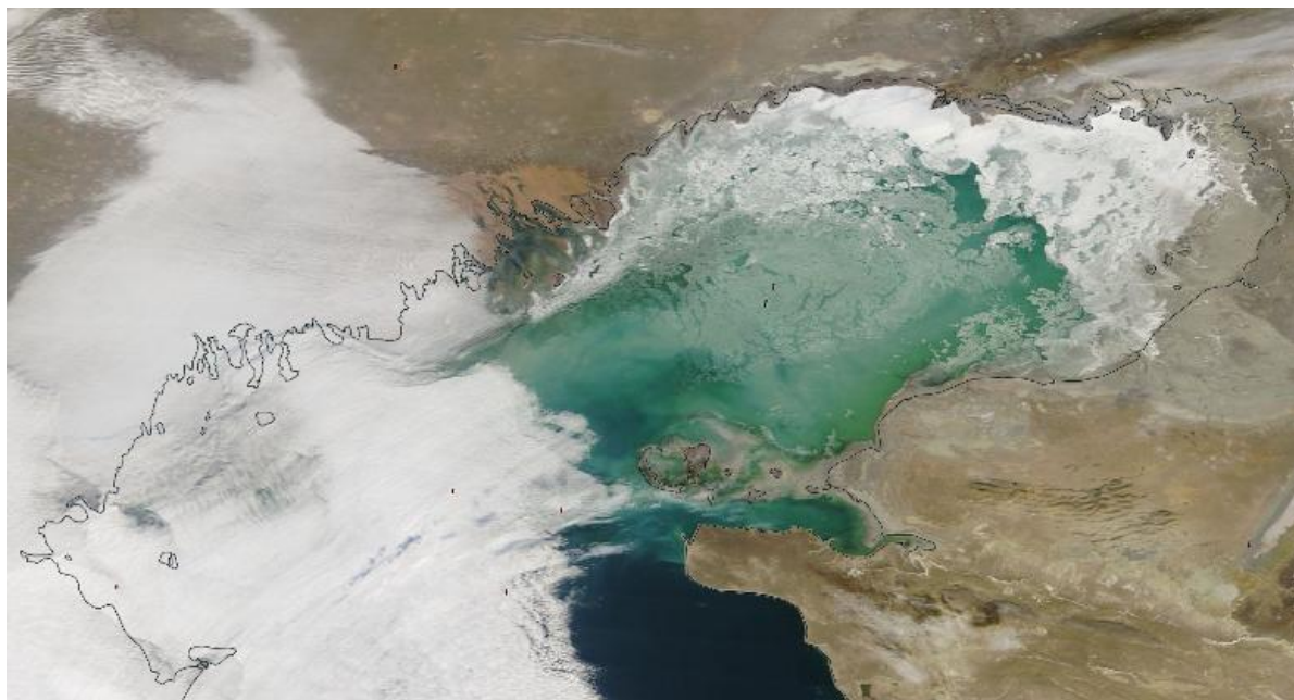
1-сурет. 2025 ж. 1 ақпан ғарыштан түсірілген Каспий теңізінің NASA/GSFC фотосуреті
