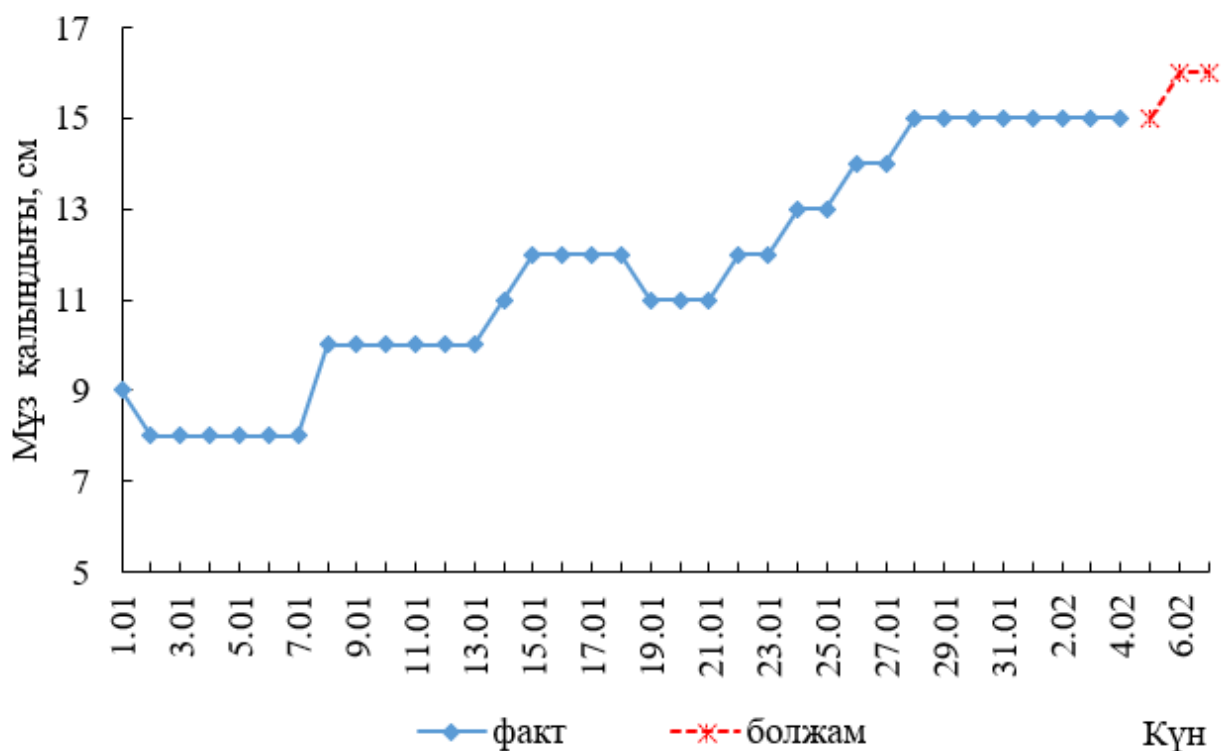
1-сурет. 2025 жылдың 1 қаңтары мен 2025 жылдың 18 ақпаны аралығында Пешной станциясының мәліметтері бойынша мұз қалыңдығының уақыт бойынша өзгерісі
