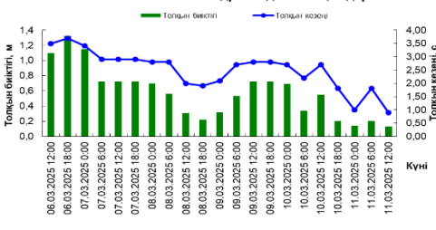
21141 квадратындағы толқындар
