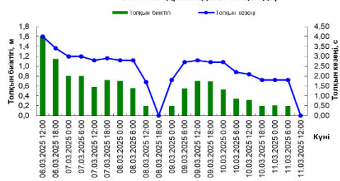
21050 квадратындағы толқындар
