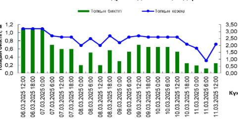
21142 квадратындағы толқындар
