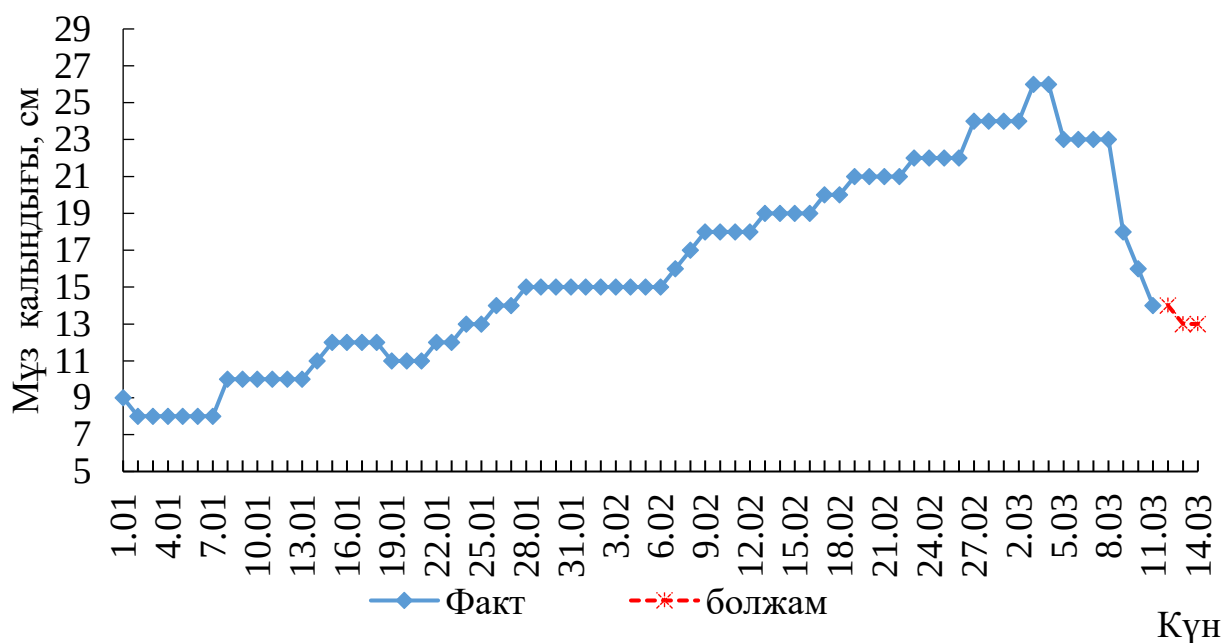
1-сурет. 2025 жылдың 1 қаңтары мен 2025 жылдың 10 наурыз аралығында Пешной станциясының мәліметтері бойынша мұз қалыңдығының уақыт бойынша өзгерісі
