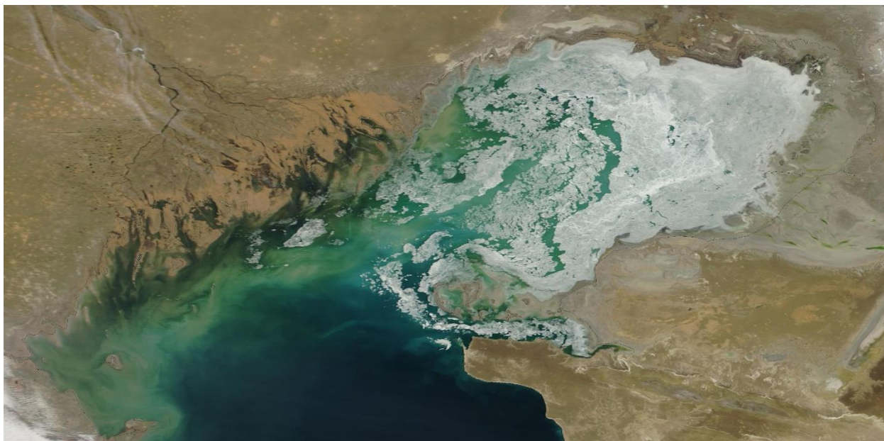
1-сурет. 2025 ж. 10 наурыз ғарыштан түсірілген Каспий теңізінің NASA/GSFC фотосуреті
