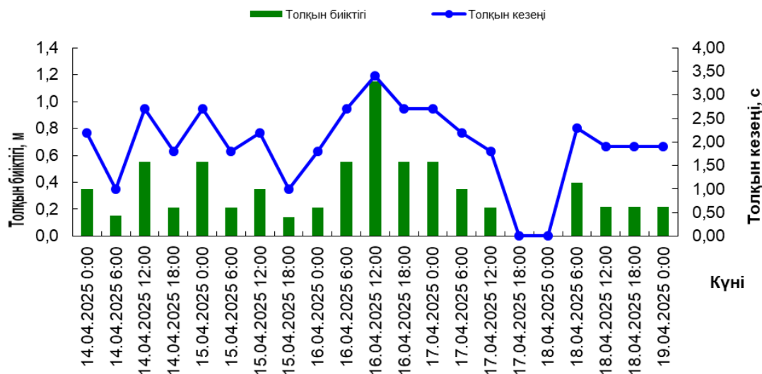
21050 квадратындағы толқындар
