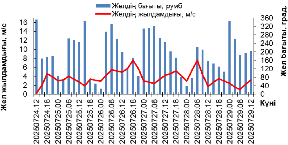
Саура ауданындағы жел жағдайлары
