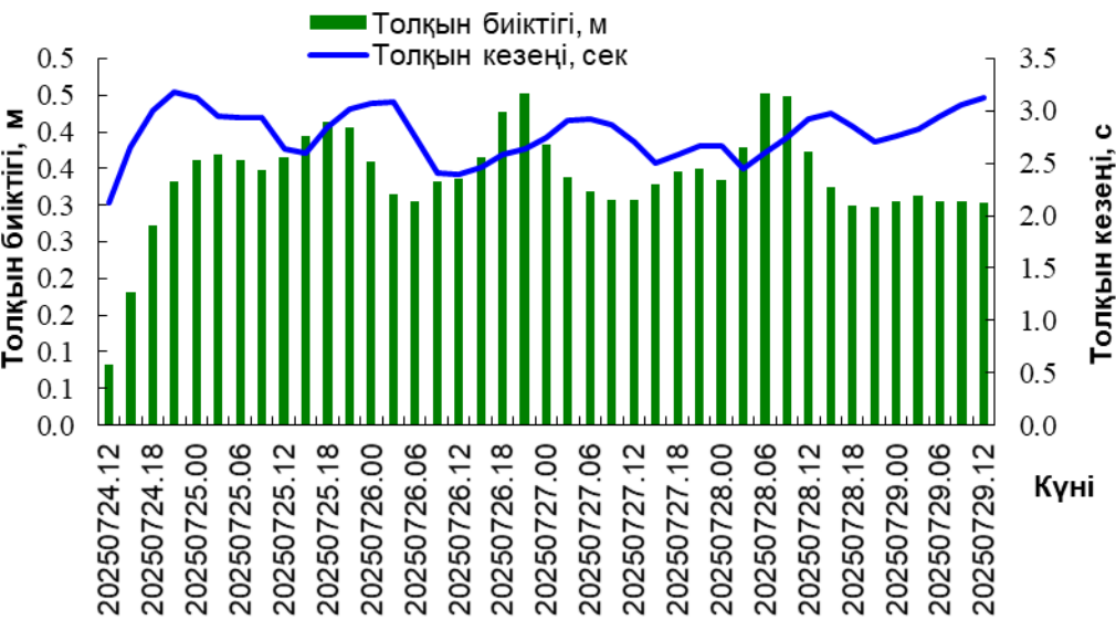
Саура ауданындағы толқындар
