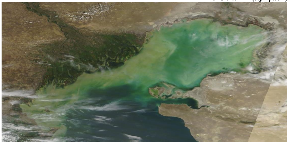
1-сурет. 2025 ж. 09 қыркүйектегі ғарыштан түсірілген Каспий теңізінің NASA/GSFC фотосуреті
