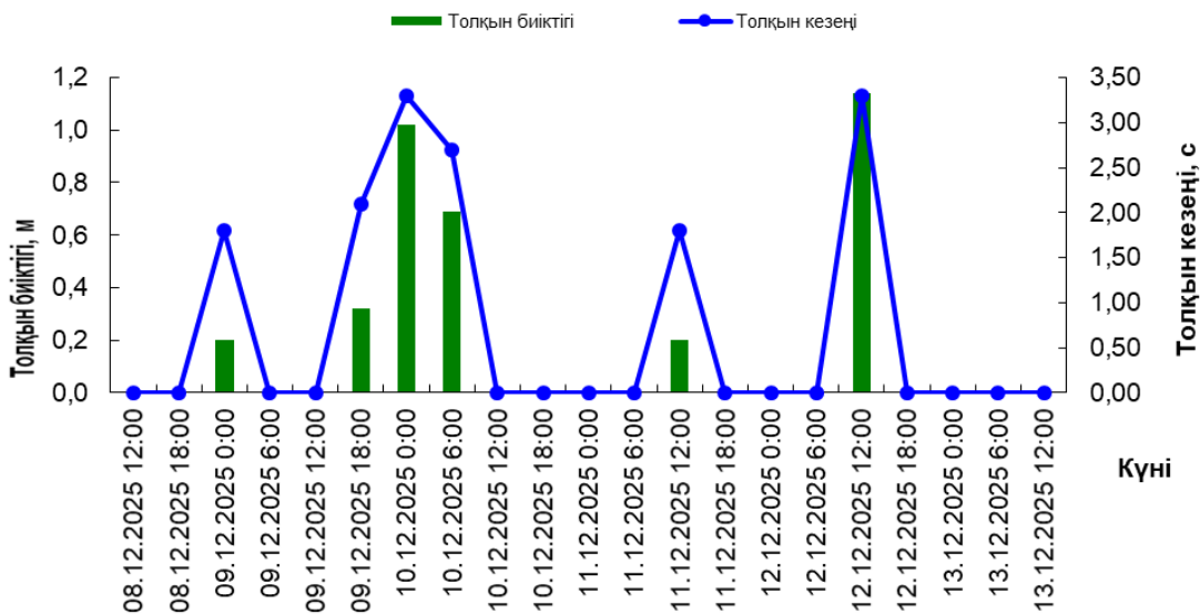
21050 квадратындағы толқындар
