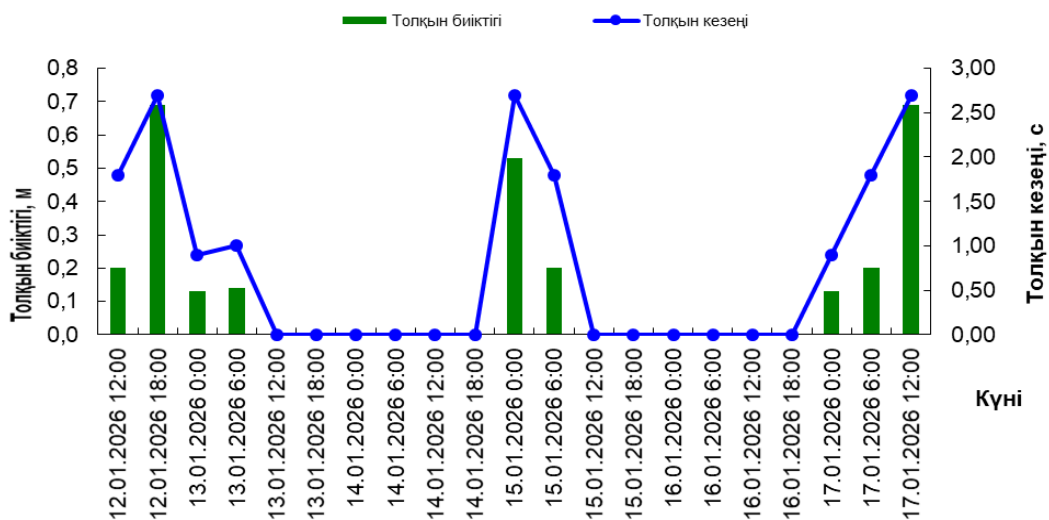
21050 квадратындағы толқындар
