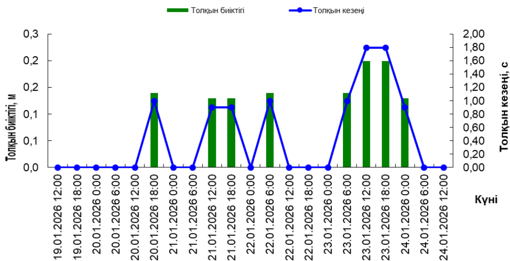
21050 квадратындағы толқындар
