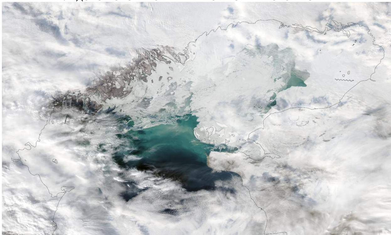
Космический снимок Каспийского моря, 02 февраля 2026 г. (NASA/GSFC)
