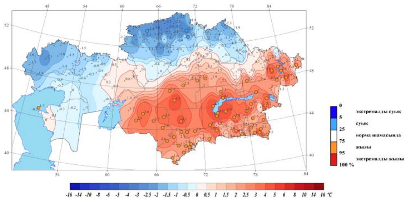
2 – сурет. 1991–2020 жылдардагы кезеңге қатысты есептелген 2026 жылғы қаңтар айындағы орташа айлық ауа температурасы (°C) аномалияларының кеңістіктік таралуы және 1941–2026 жылдардагы кезеңге сәйкес есептелген ауа температурасының аспау ықтималдығының кеңістіктік таралуы
