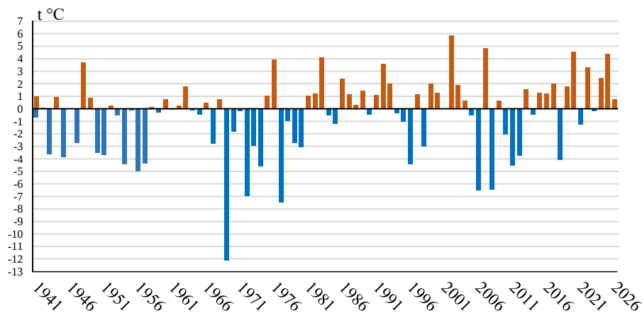
1-сурет. 1941-2026 жылдар кезеңінде Қазақстан аумағы бойынша орташаланған жылдық ауа температурасы ( ^{\circ}\text{C} ) ауытқуларының уақыттық қатарлары.
